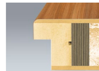
Konstrukce hrany Classen Hard profil PF / Konštrukcia hrany Classen Hard profil PF
