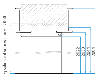
▲ OŚCIEŻNICA REGULOWANA
