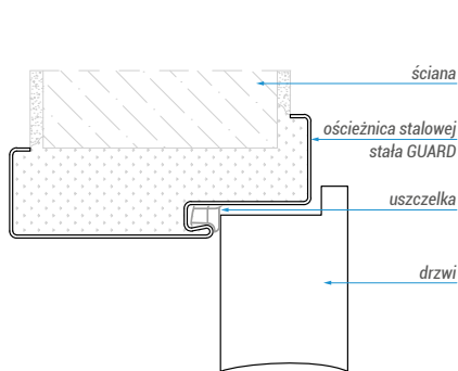
▲ OŚCIEŻNICA GUARD STAŁA STAŁA
