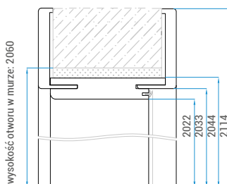
▼ OŚCIEŻNICA REGULOWANA 80 NOWOŚĆ
