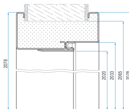
Dimensions of GUARD fixed door frame [mm]: Размеры фиксированной коробки GUARD [mm]:
