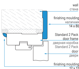
14x80 moulding can be also installed as a wall base moulding 14x80 планка 14x80мм как наличник а также плинтус
