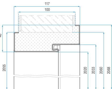
Dimensions of FIRE wooden door frame [mm]: Размеры деревянной противопожарной коробки [мм]:
