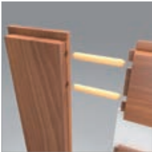
Frame construction Рамовая конструкция
